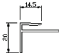
DE 898 3mm F-Section
